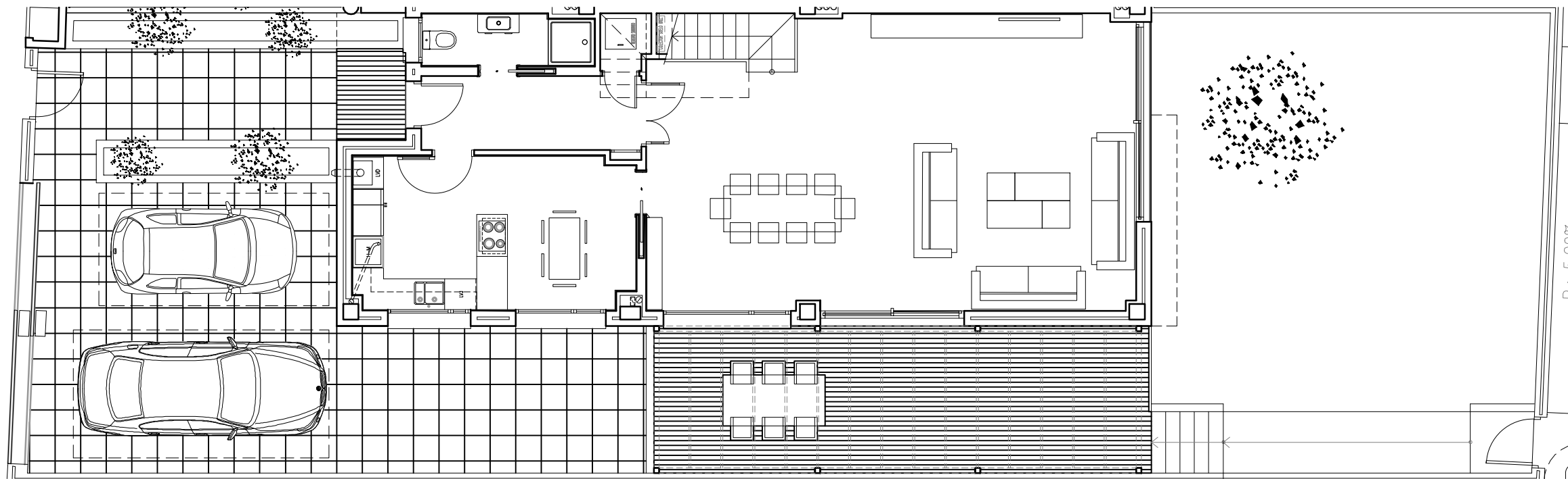
PLANTA BAJA
