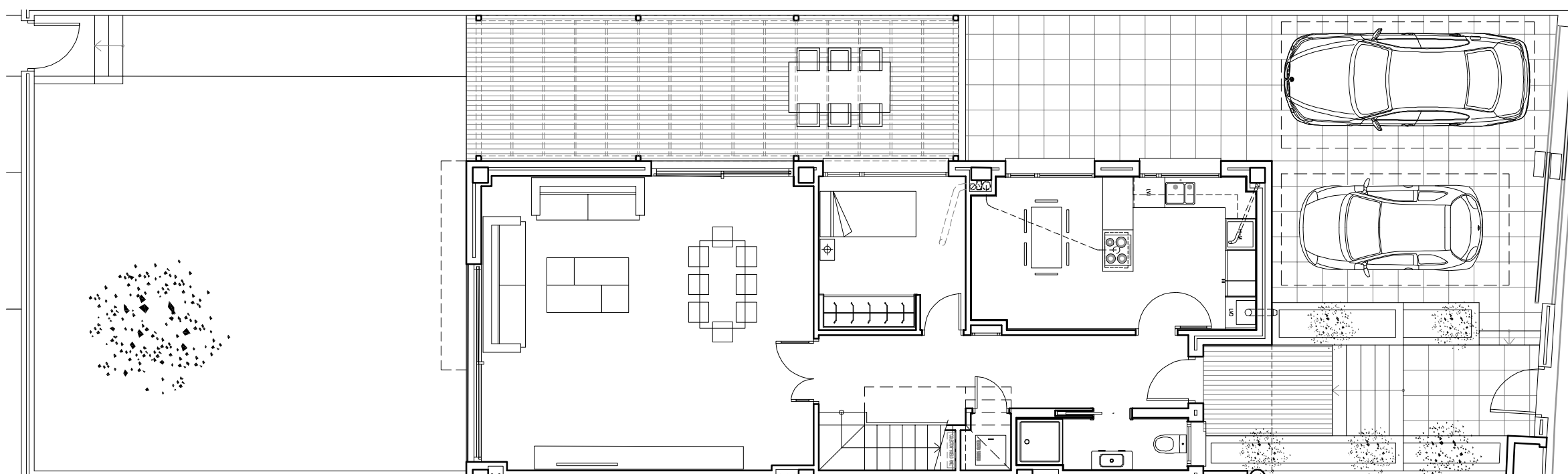
PLANTA BAJA
