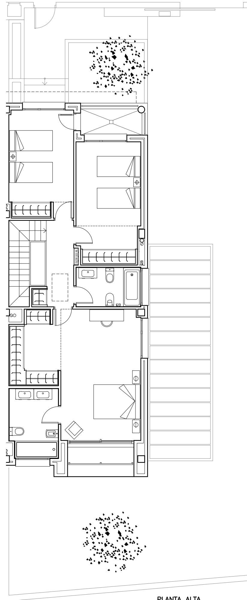
PLANTA ALTA
