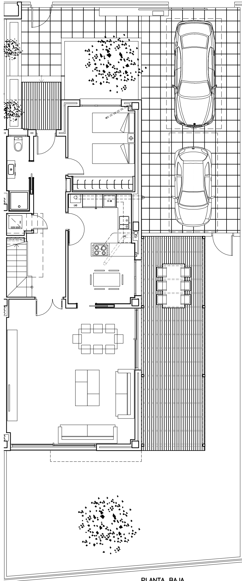
PLANTA BAJA
