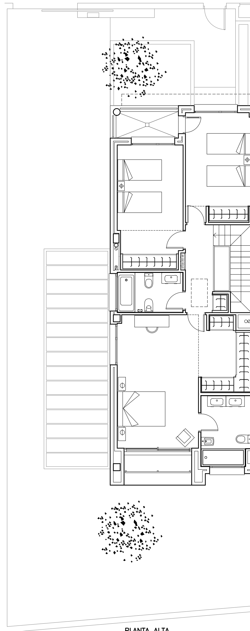
PLANTA ALTA
