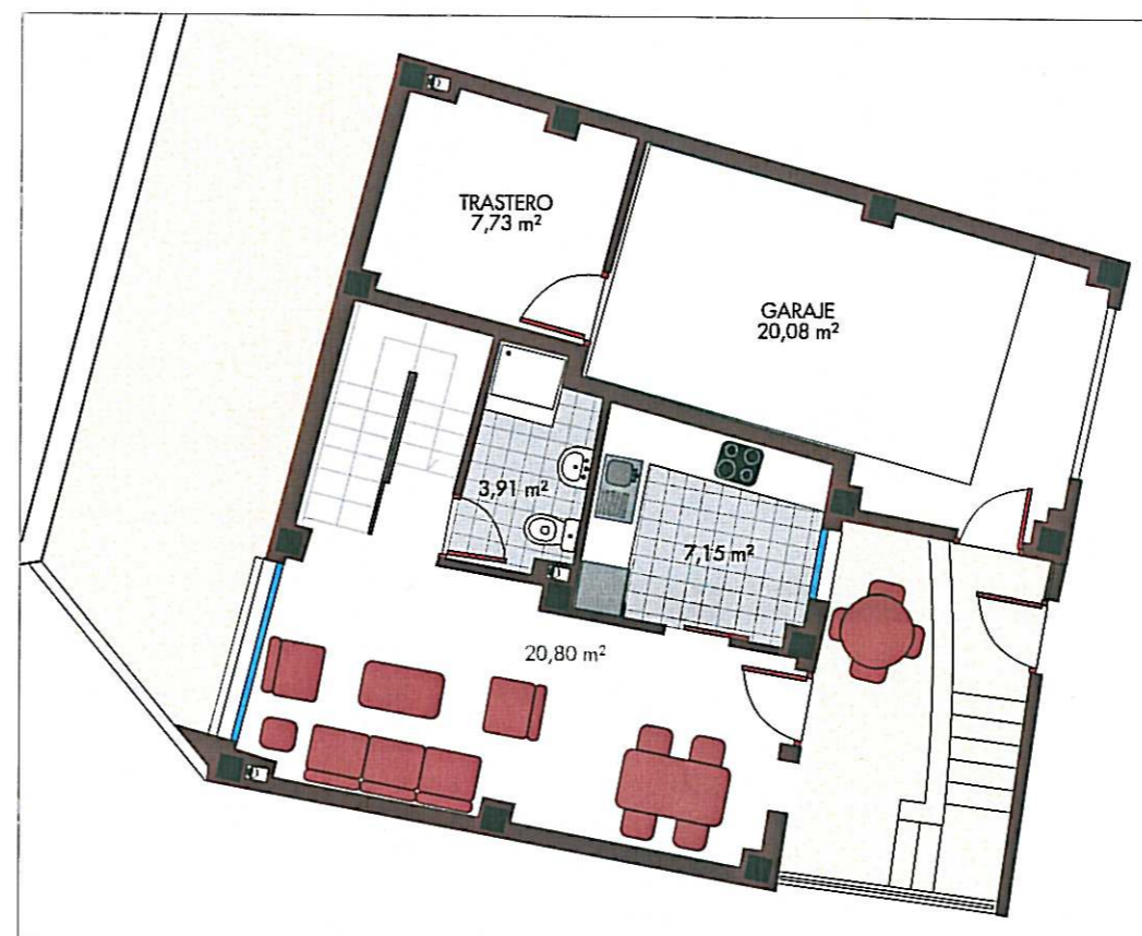
Planta Baja
