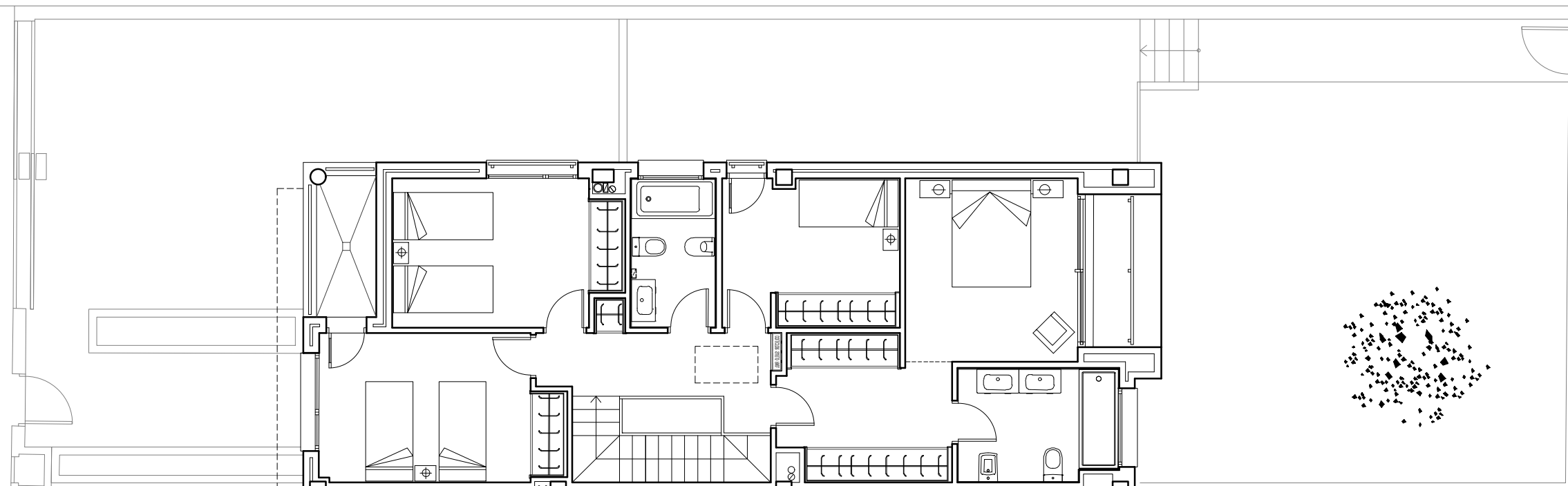
PLANTA ALTA
