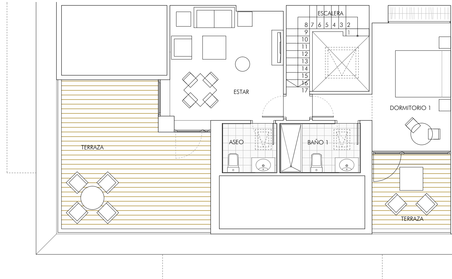
DÚPLEX. PLANTA ÁTICO
