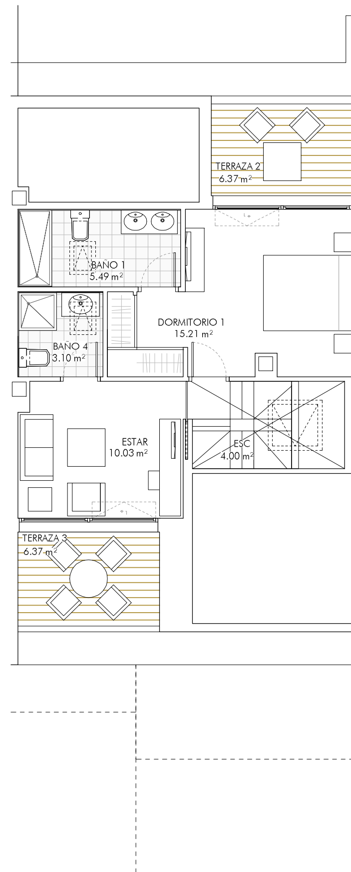
DÚPLEX. PLANTA ÁTICO
