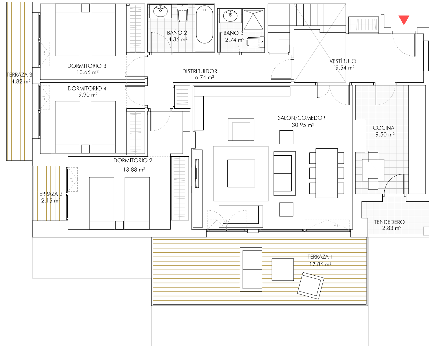
DÚPLEX. PLANTA ACCESO
