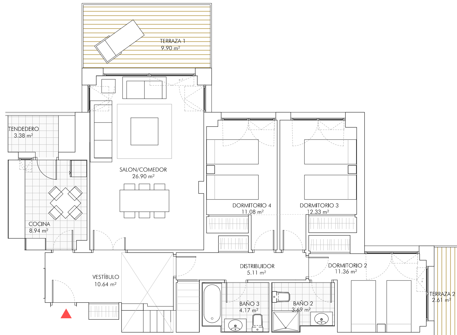
DÚPLEX. PLANTA ACCESO
