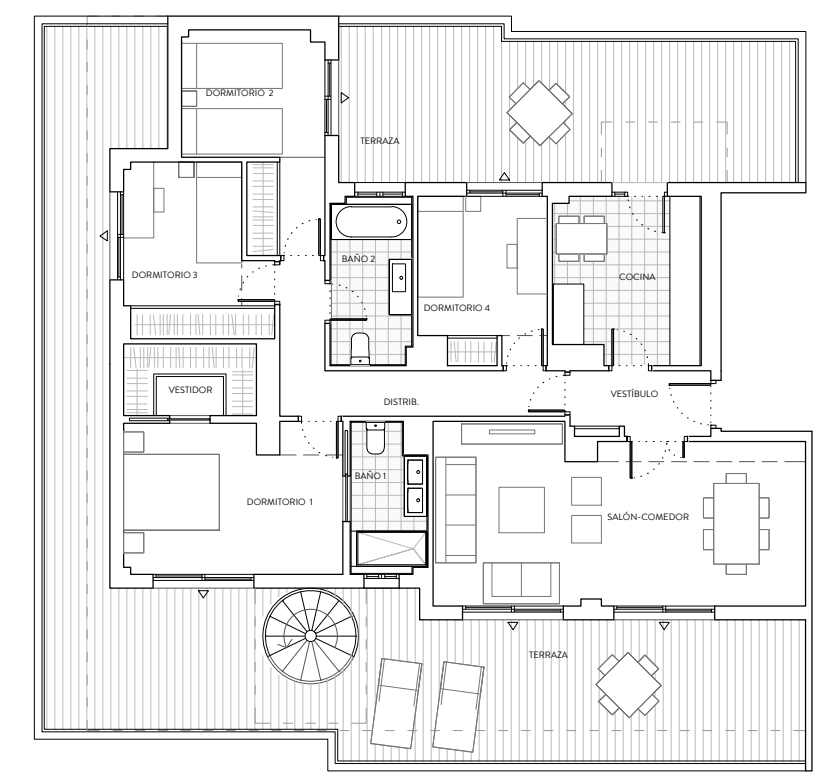
PLANTA TERRAZAS ESCALA 1:150
