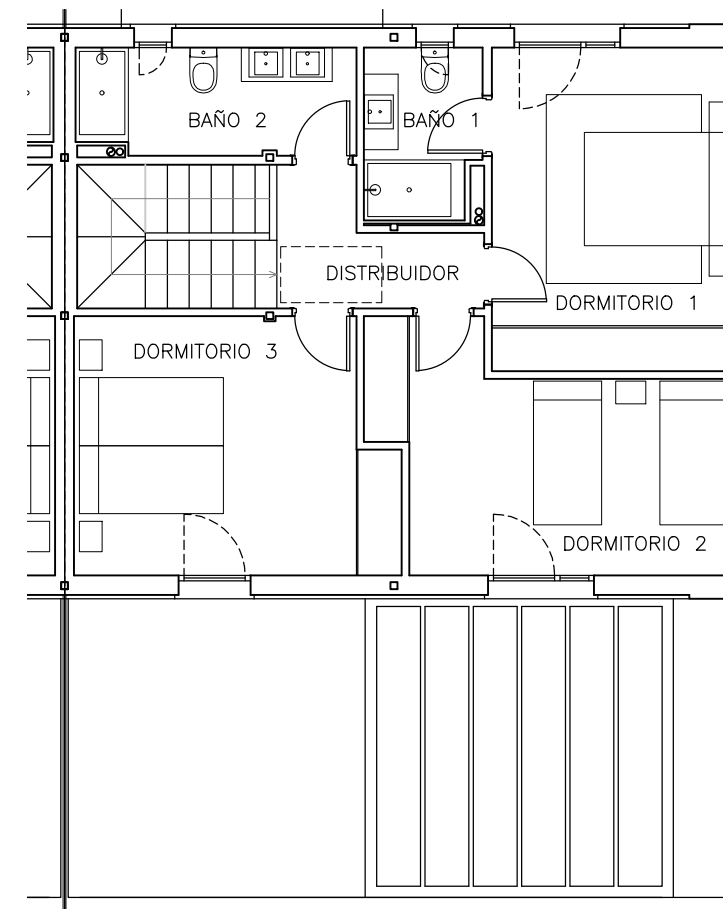
PLANTA ALTA
