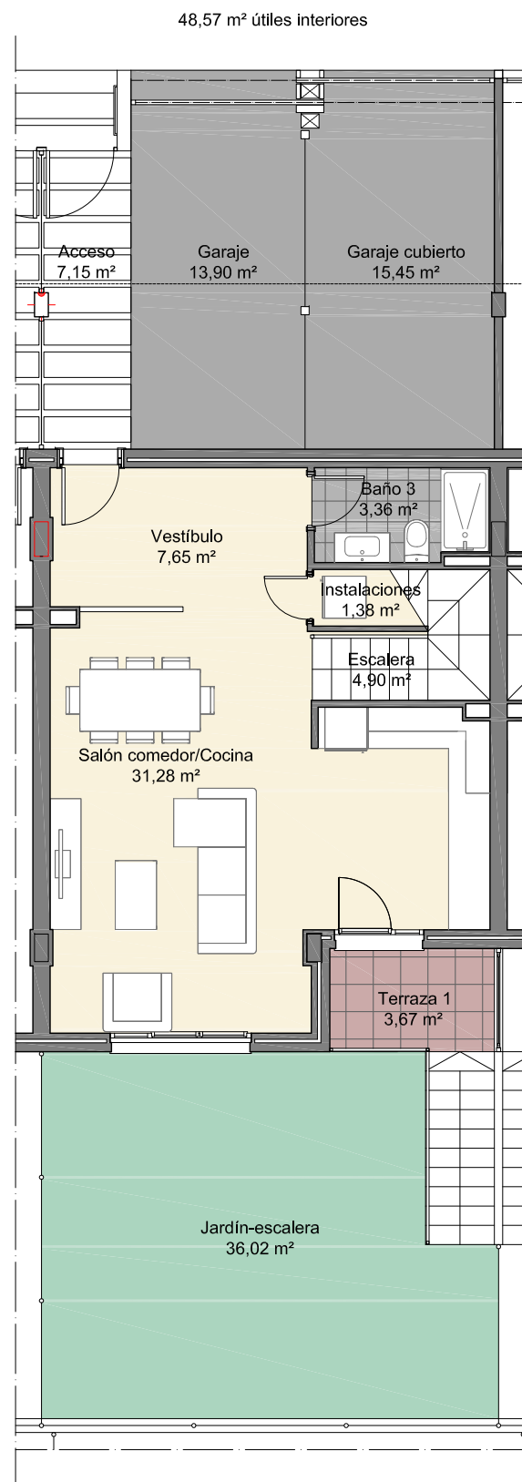
PLANTA BAJA
