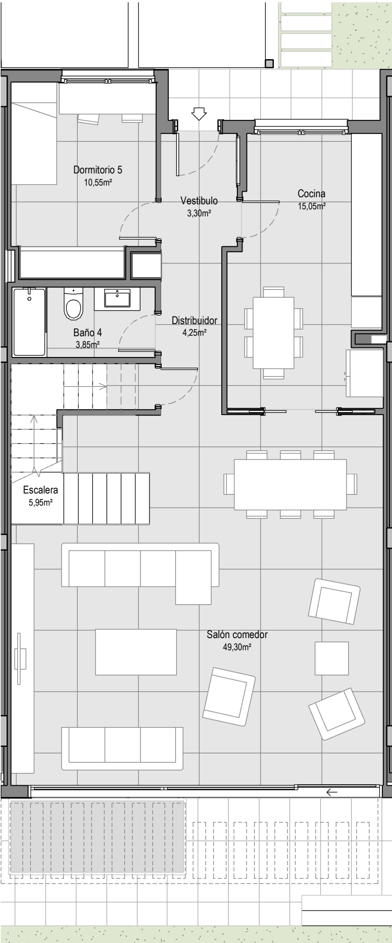
Planta baja
