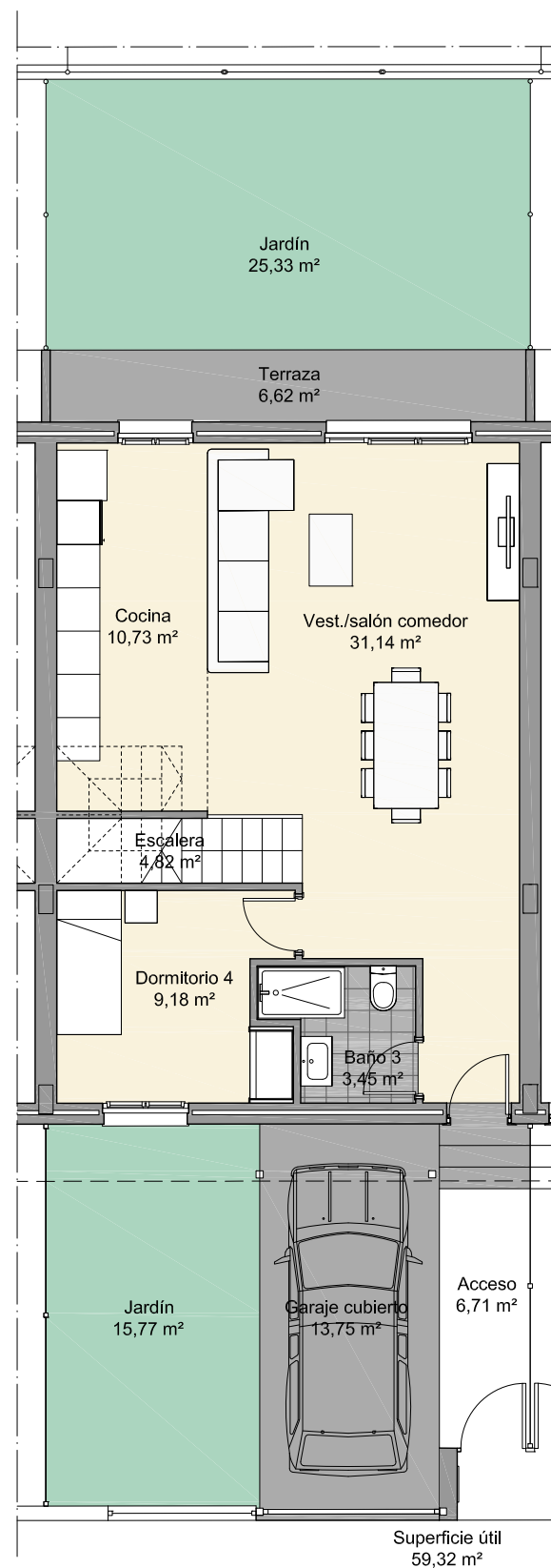
PLANTA BAJA
