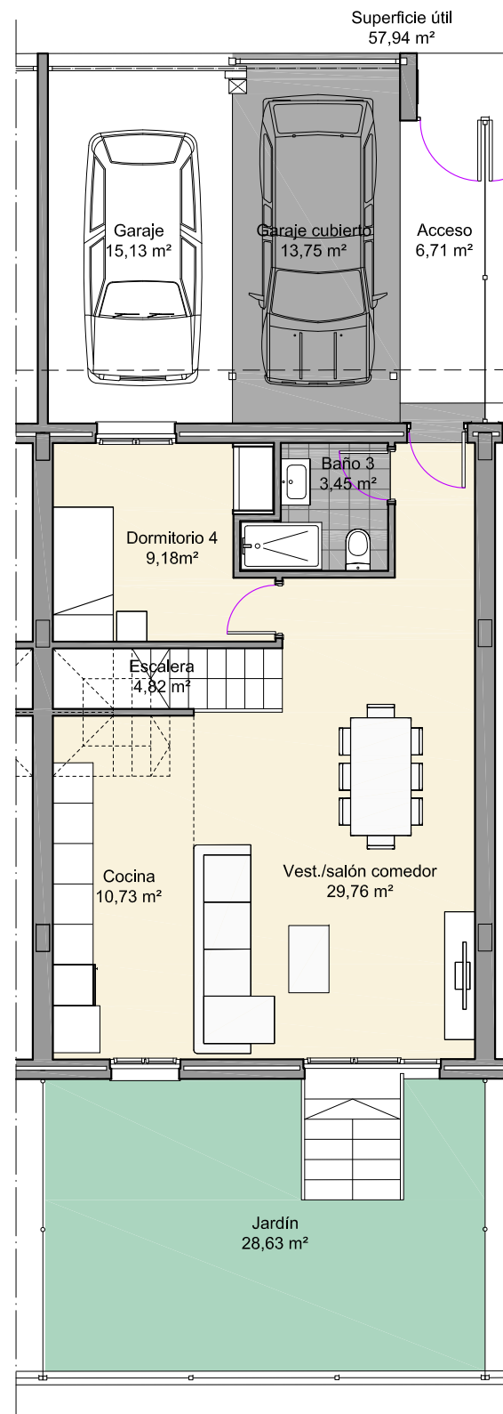
PLANTA BAJA
