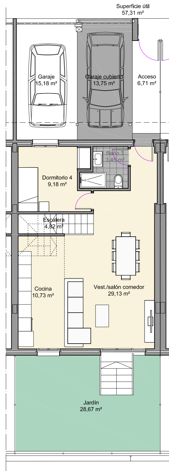
PLANTA BAJA
