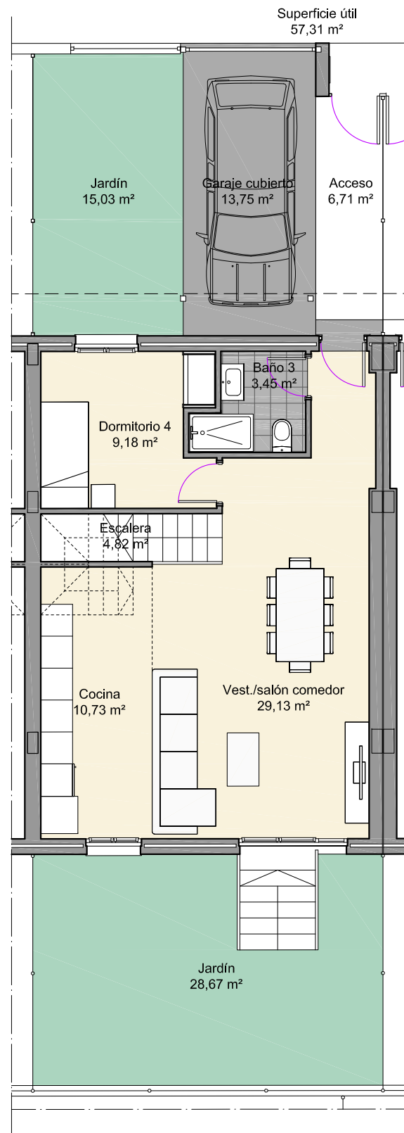
PLANTA BAJA
