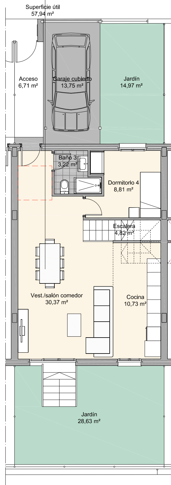
PLANTA BAJA
