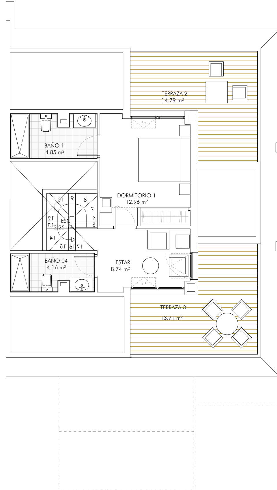
DÚPLEX. PLANTA ÁTICO
